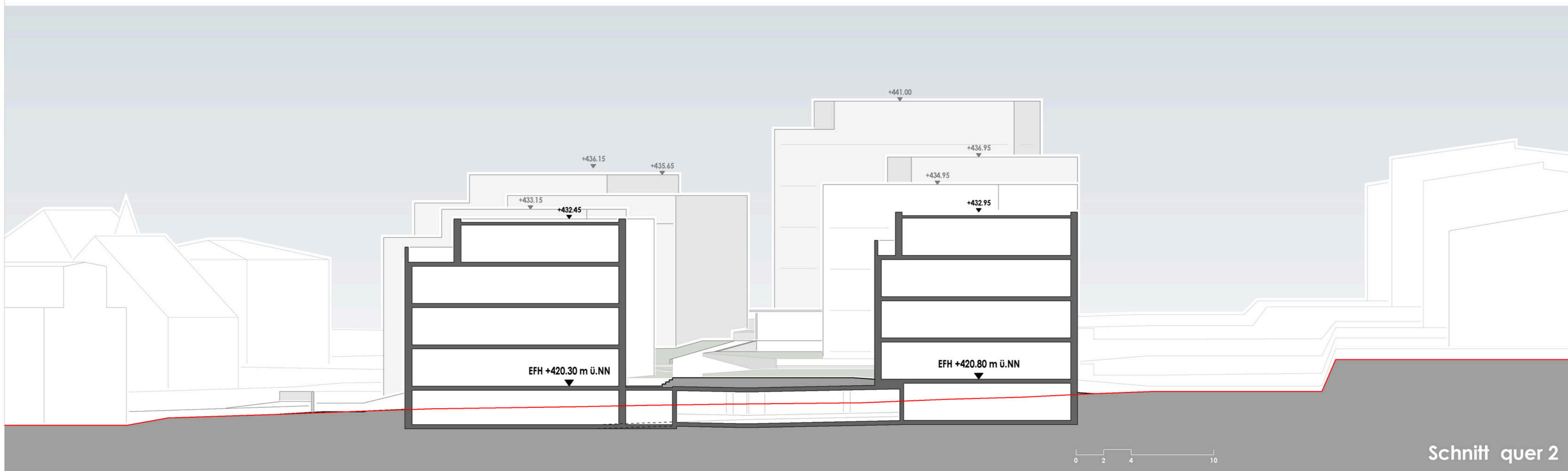
Schnitt quer 1
