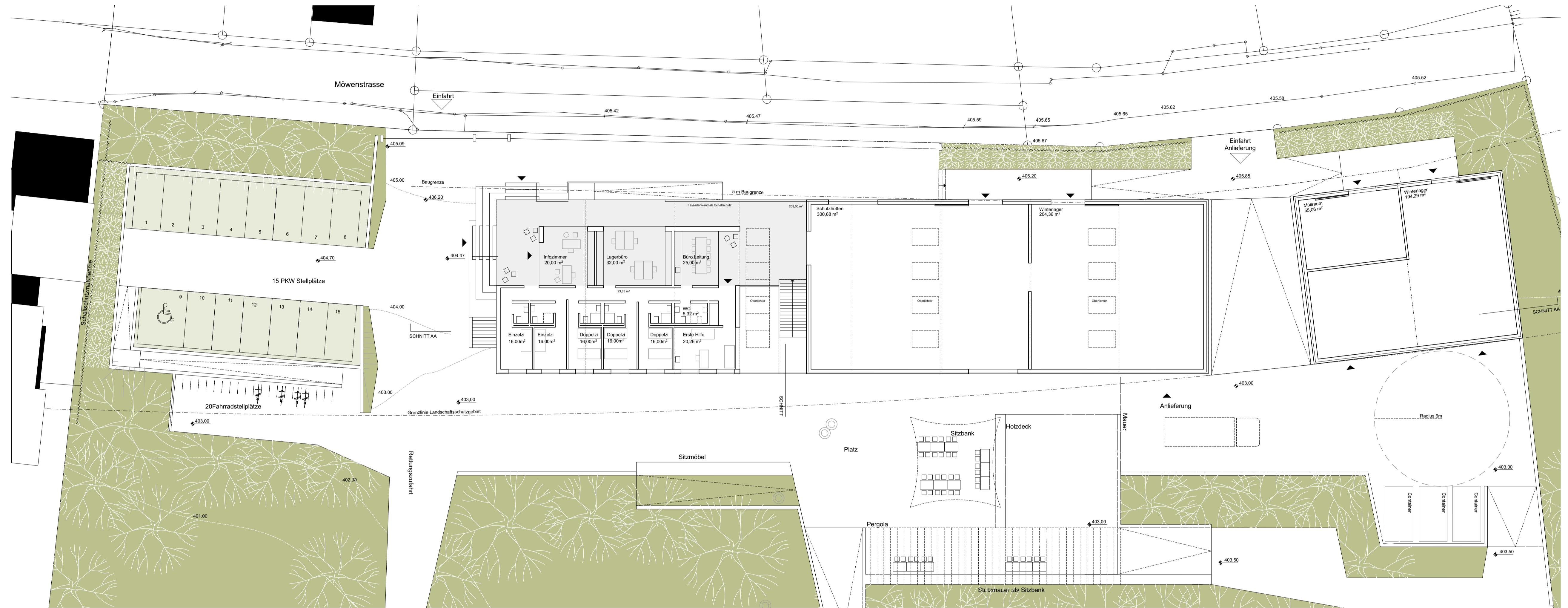
GRUNDRISS ERDGESCHOSS 1:200
