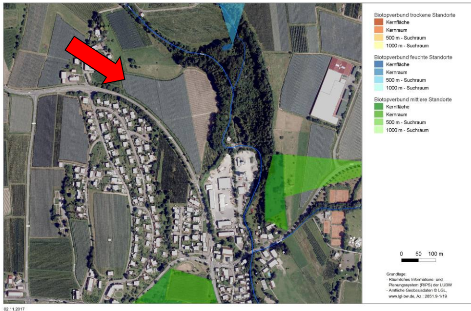
Schutzgebiete
