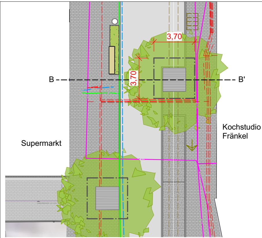
Lageplan M 1:200
