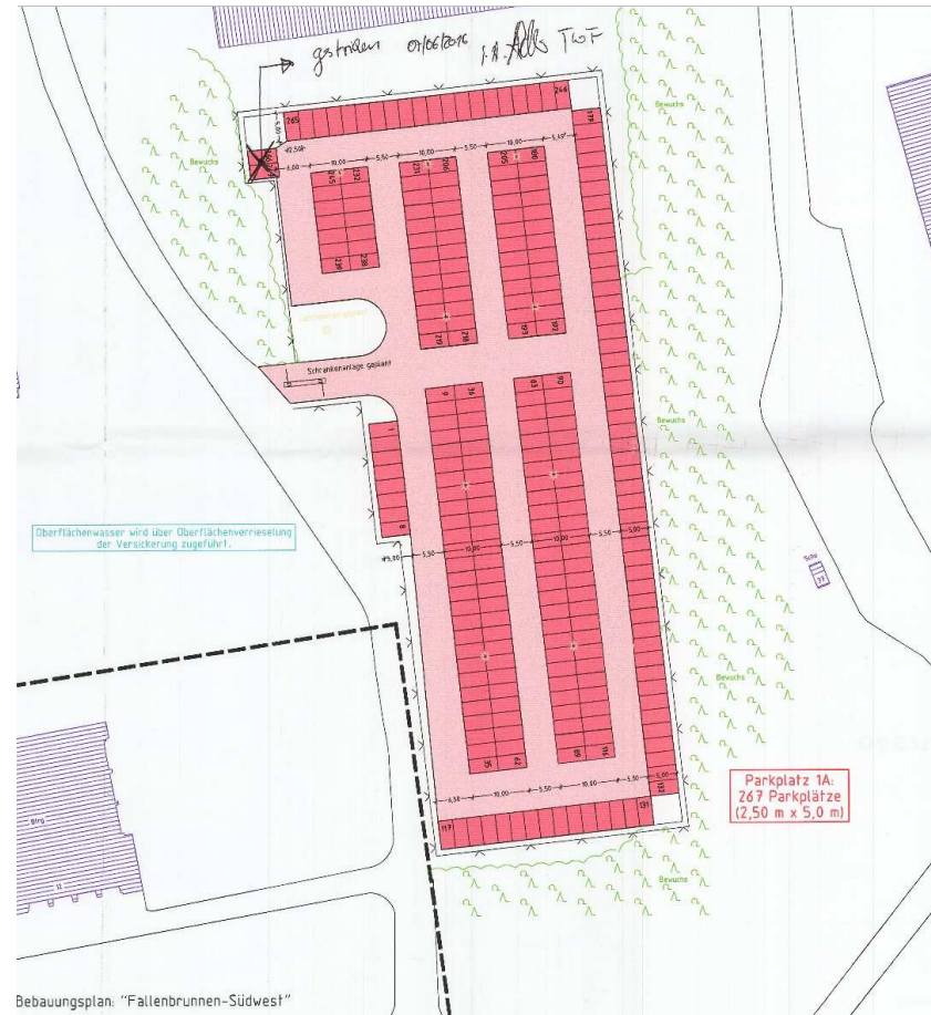
Lageplan Ersatzparkplatz DHBW (ehemals Fallbrunnen 11; Planvorlage SWSee)
