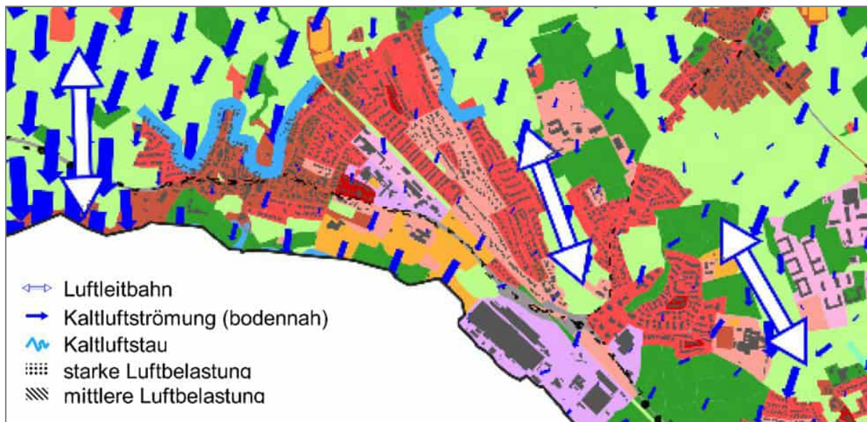
Abb. 24: Auszug aus der Klimatopkarte
