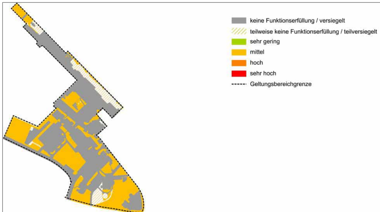
Abb. 14: Bewertung der Bodenfunktionen im Geltungsbereich
