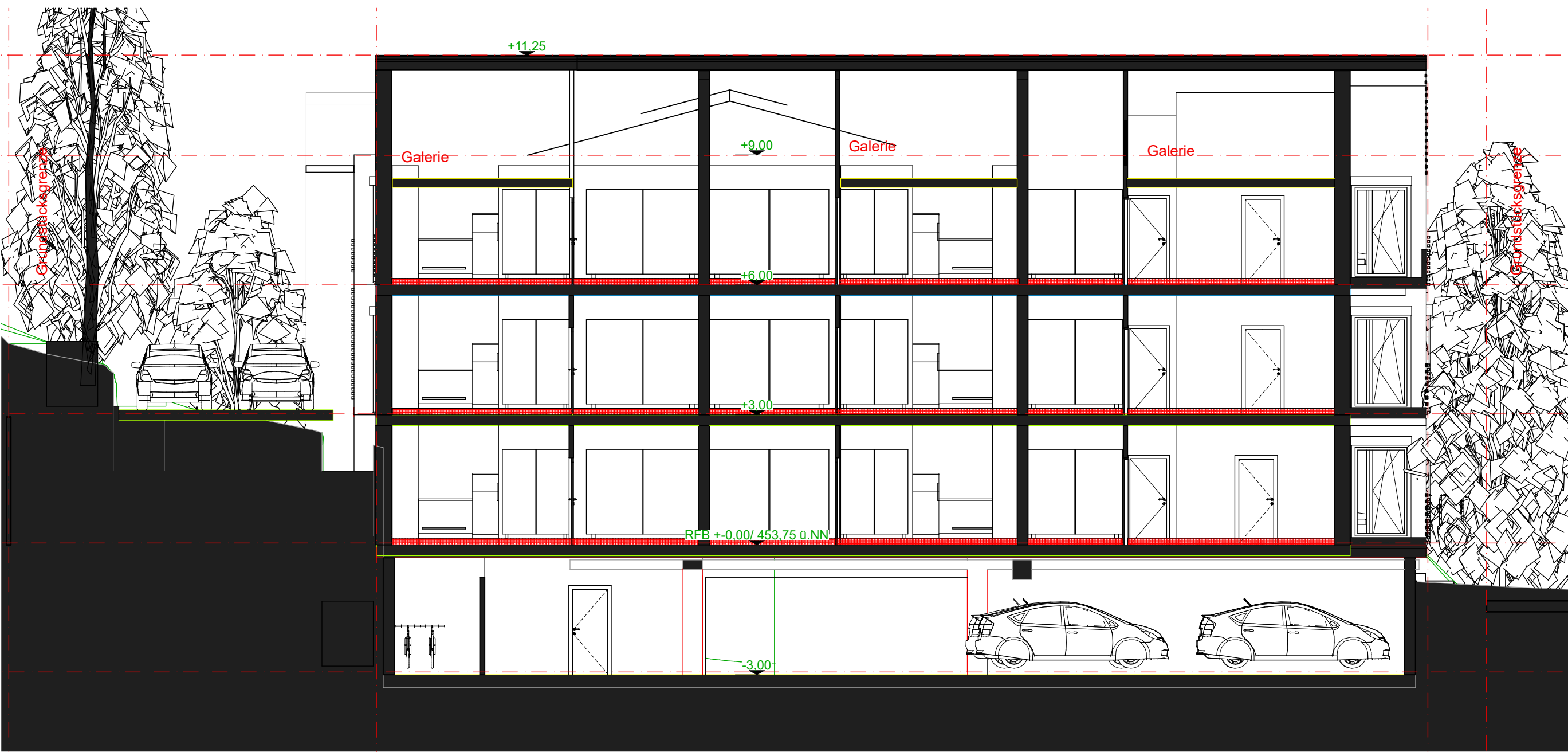
Längsschnitt Gebäude West
