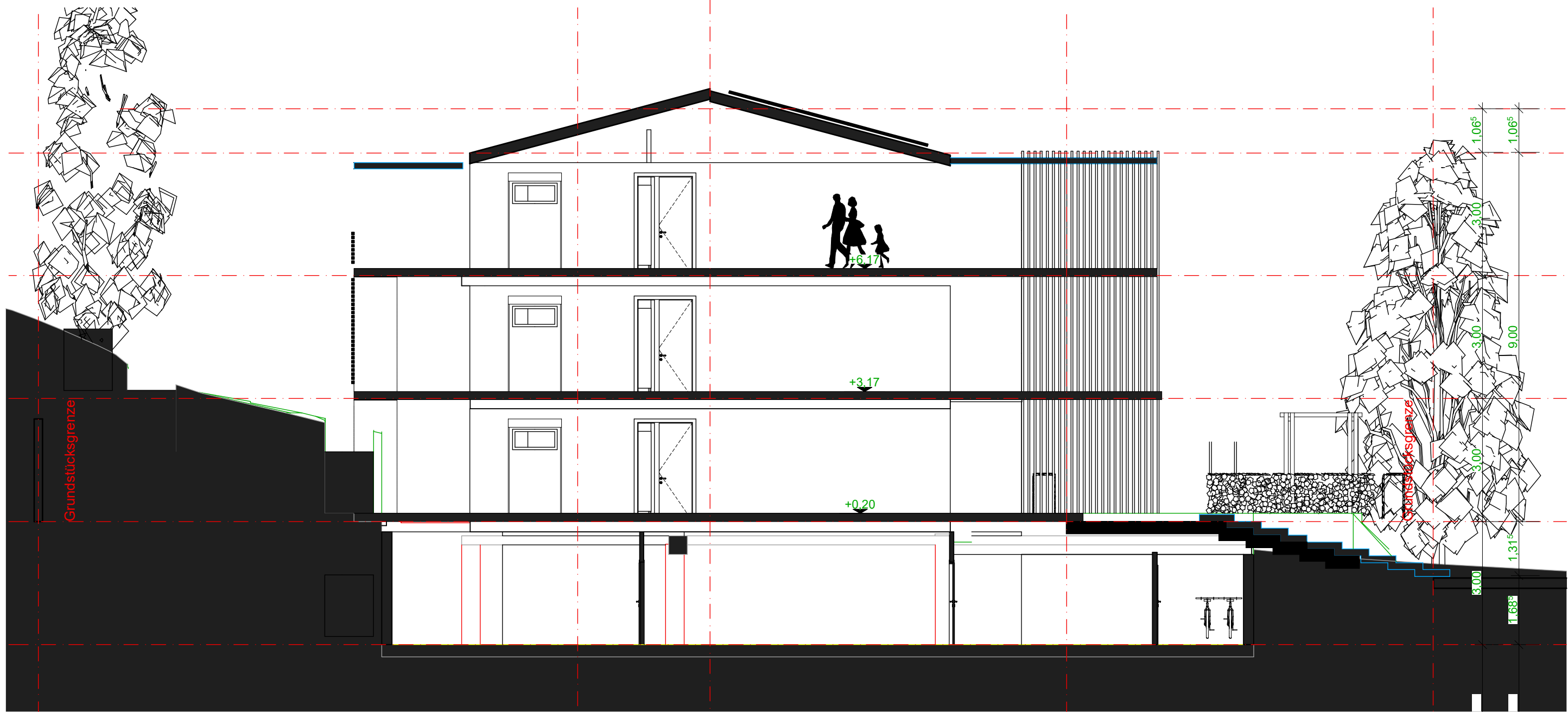
Schnitt Laubengang Gebäude Mitte
