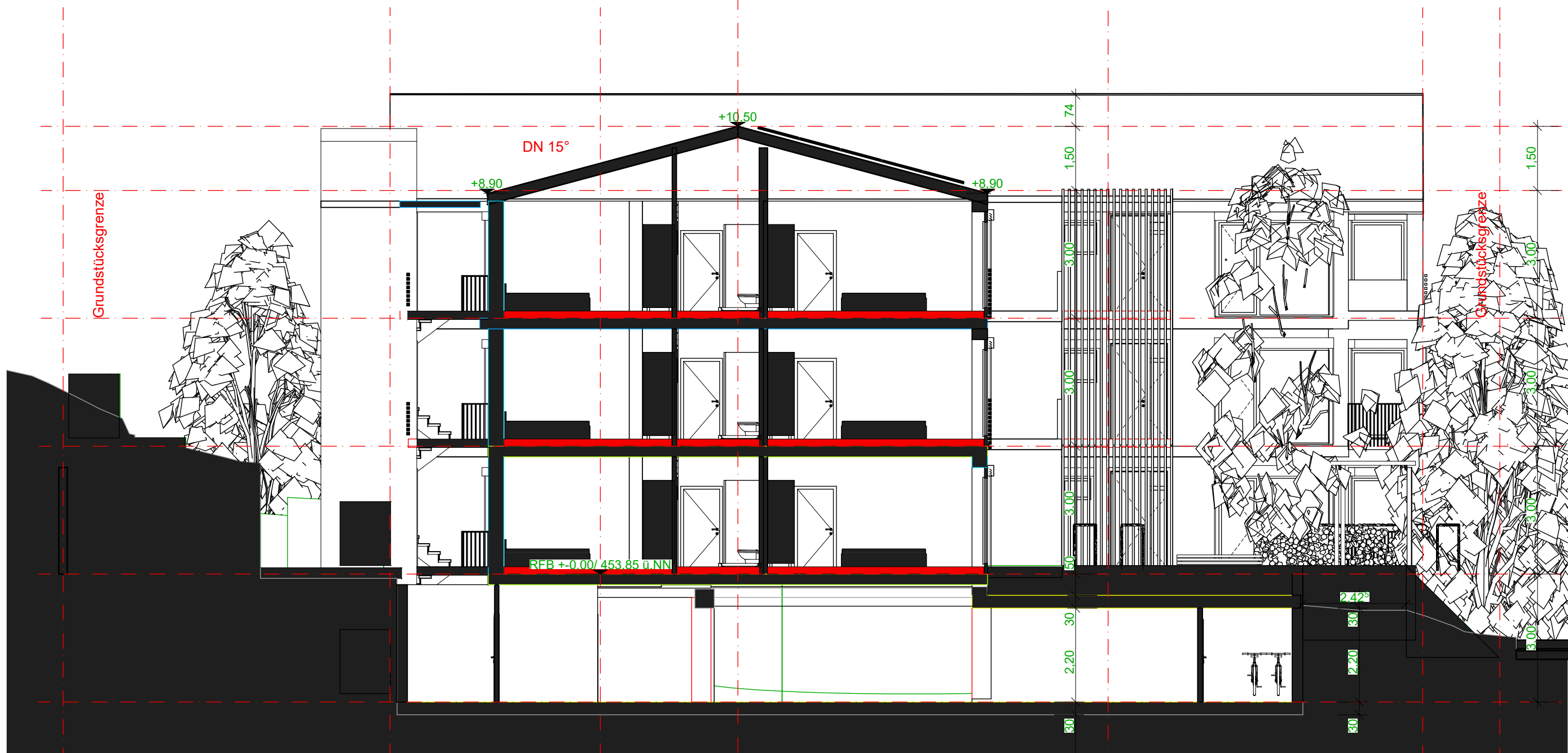
Schnitt Gebäude Mitte
