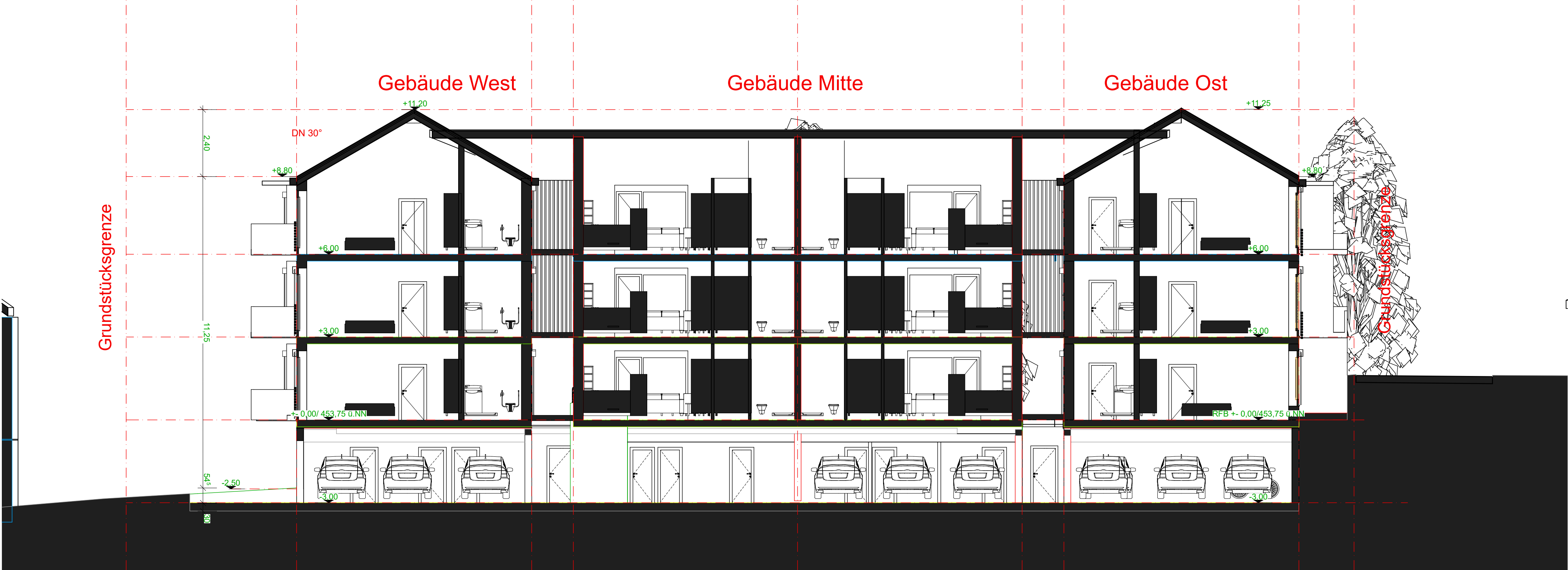
Querschnitt
