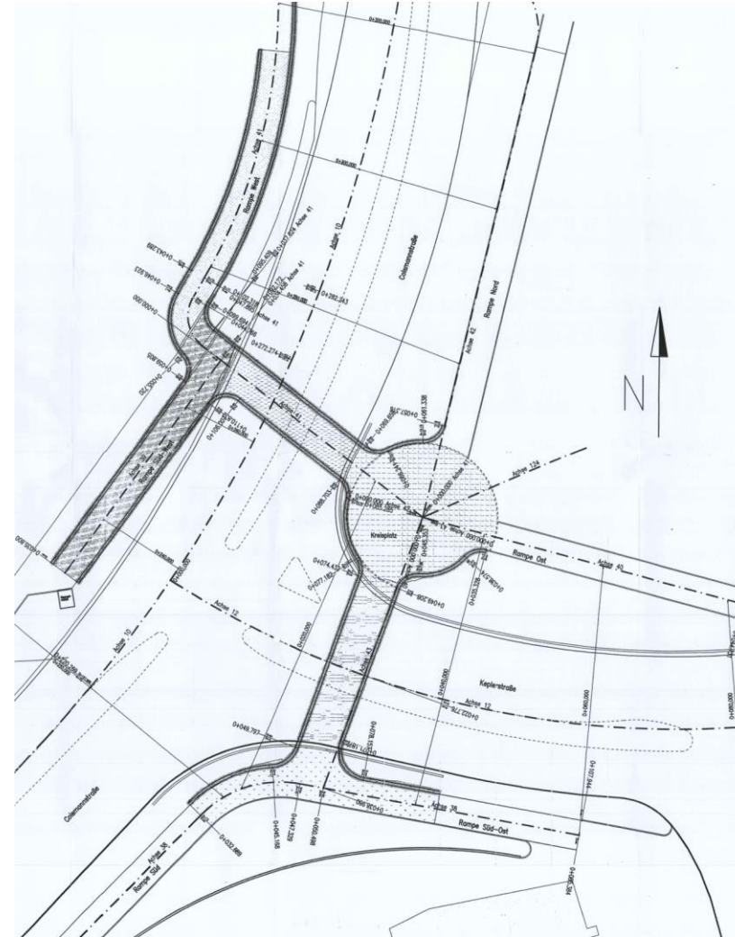
Übersichtsplan des Unterführungsbauwerkes Maybachplatz
